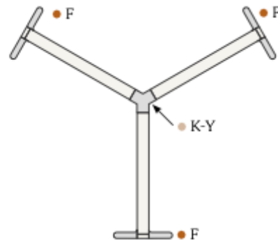
EXEMPEL (Koppling Y-120°)
